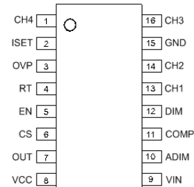
SO-16
