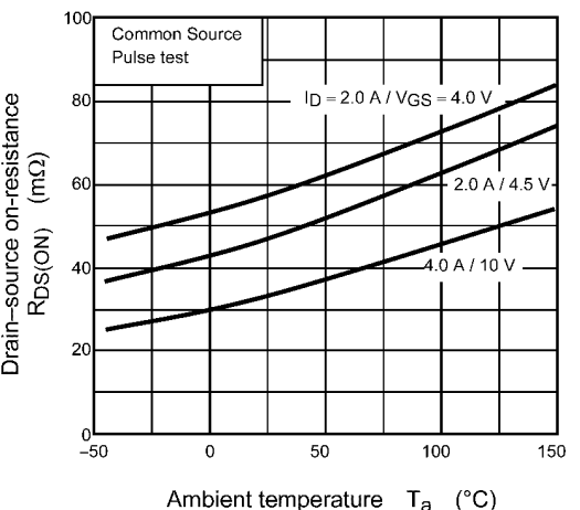
Fig. 9.6 R_{DS(ON)} - T_a
