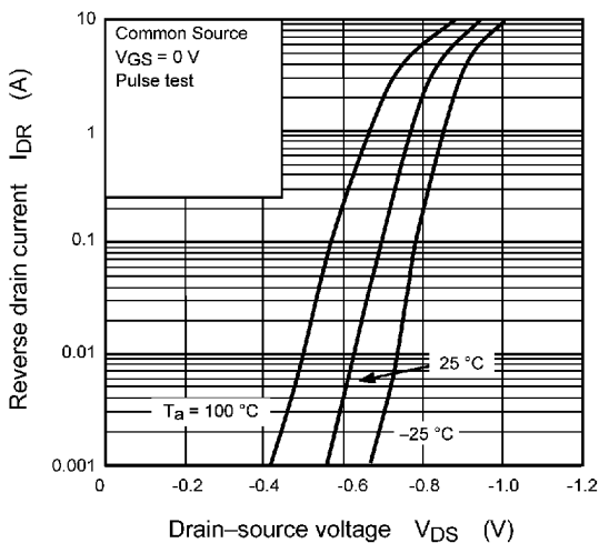
Fig. 9.9 I_{DR} - V_{DS}
