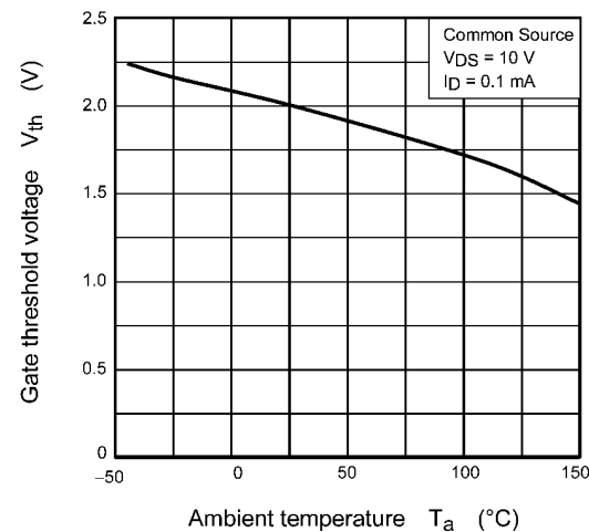
Fig. 9.7 V_{th} - T_a
