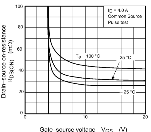
Fig. 9.4 R_{DS(ON)} - V_{GS}
