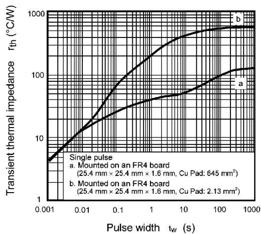
Fig. 9.13 r_{th} - t_w
