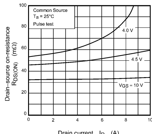
Fig. 9.5 R_{DS(ON)} - I_D
