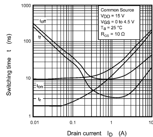
Fig. 9.11 t - I_D
