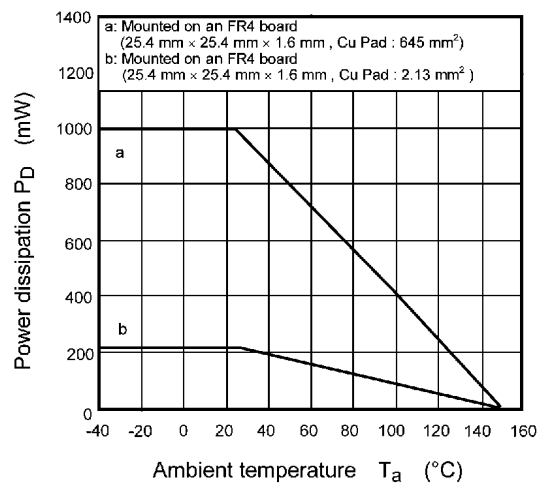
Fig. 9.14 P_D - T_a
