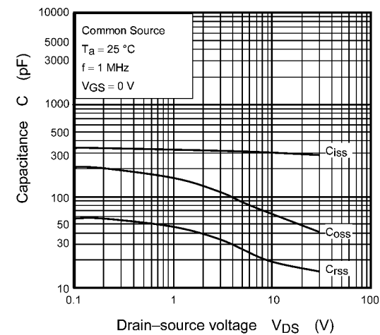
Fig. 9.10 C - V_{DS}
