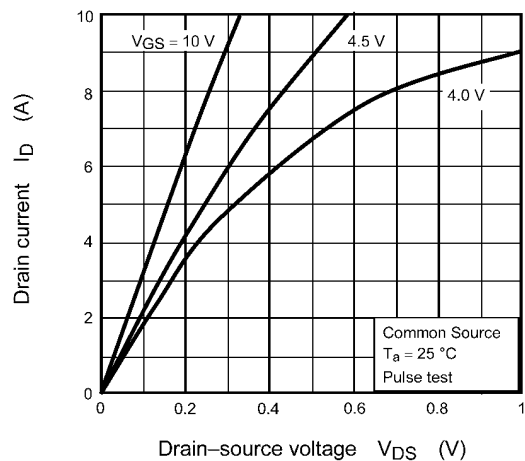
Fig. 9.1 I_D - V_{DS}
