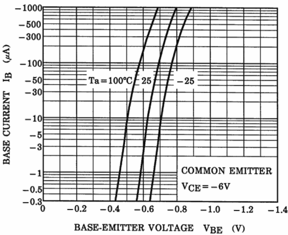
Fig. 8.2 IB - VBE
