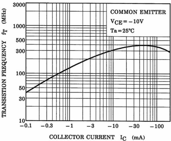
Fig. 8.4 fT - IC
