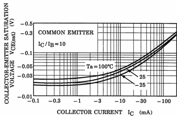
Fig. 8.5 VCE(sat) - IC
