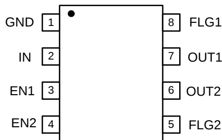
SO-8
