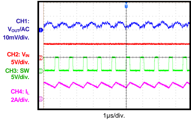
Ripple I_{OUT} = 2A
