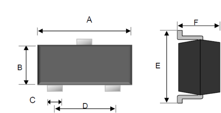
SOT-723
