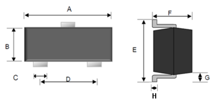
SOT-23
