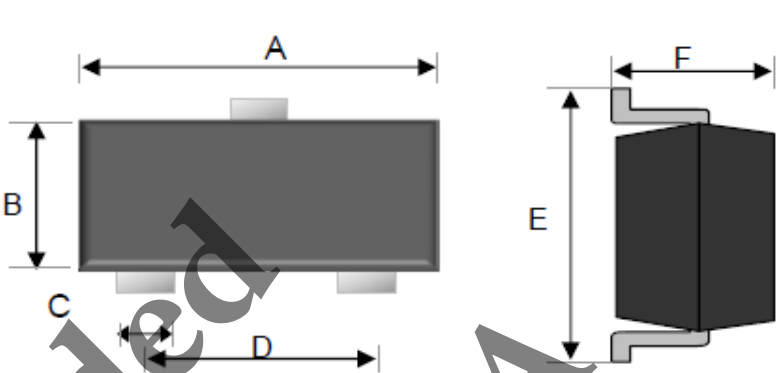
SOT-323
