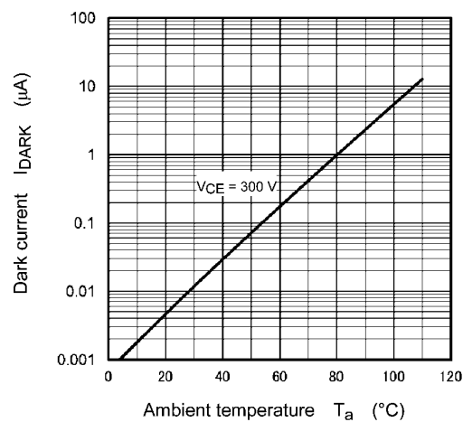
Fig. 11.11 I_{DARK} - T_a
