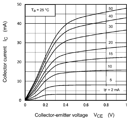
Fig. 11.8 I_C - V_{CE}
