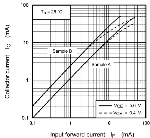
Fig. 11.9 I_C - I_F
