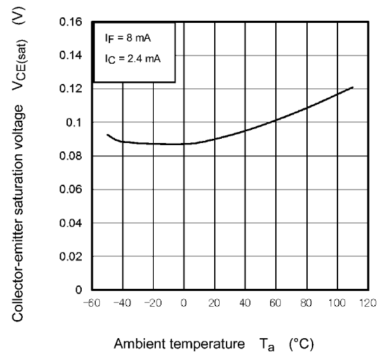
Fig. 11.12 V_{CE(sat)} - T_a
