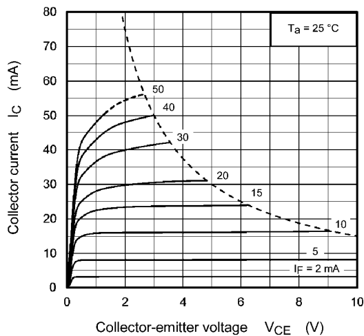
Fig. 11.7 I_C - V_{CE}
