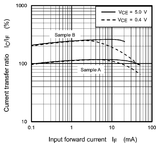
Fig. 11.10 I_C/I_F - I_F
