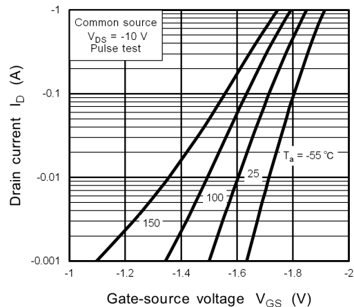
Fig. 8.7 I_D - V_{GS}
