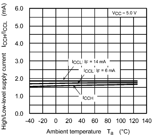
Fig. 12.2.6 I_{CCH} / I_{CCL} - T_a
