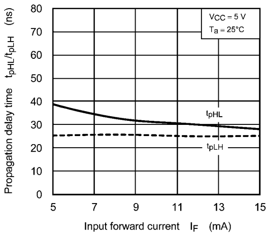
Fig. 12.2.15 t_{pHL}/t_{pLH} - I_F
