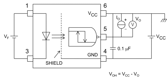
Fig. 12.1.2 V_{OH} Test Circuit
