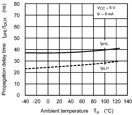
Fig. 12.2.11 t_{pHL}/t_{pLH} - T_a
