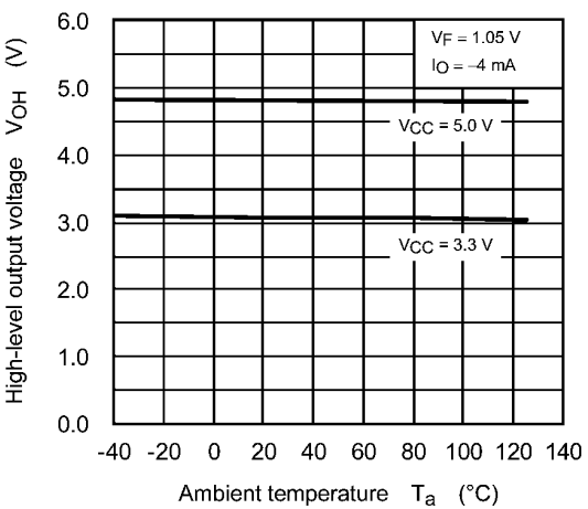
Fig. 12.2.4 V_{OH} - T_a
