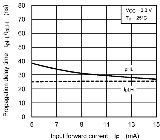
Fig. 12.2.13 t_{pHL}/t_{pLH} - I_F
