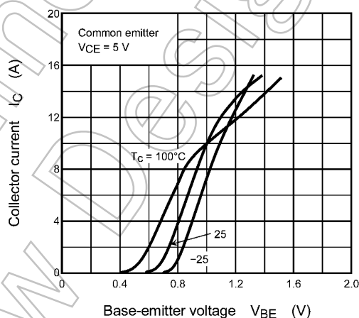
Fig. 8.4 I_c - V_{be}
