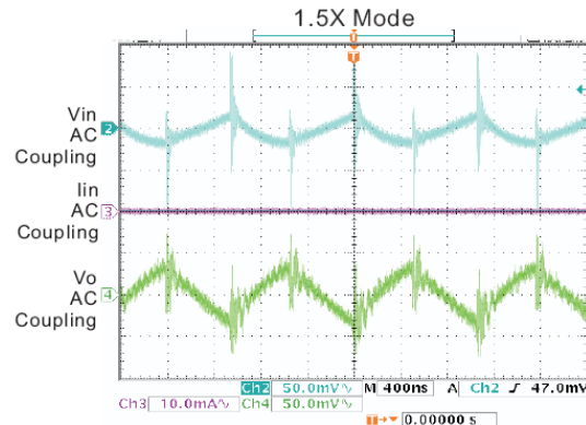
13. Output Ripple
