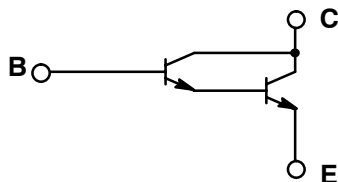
NTE273 Schematic
