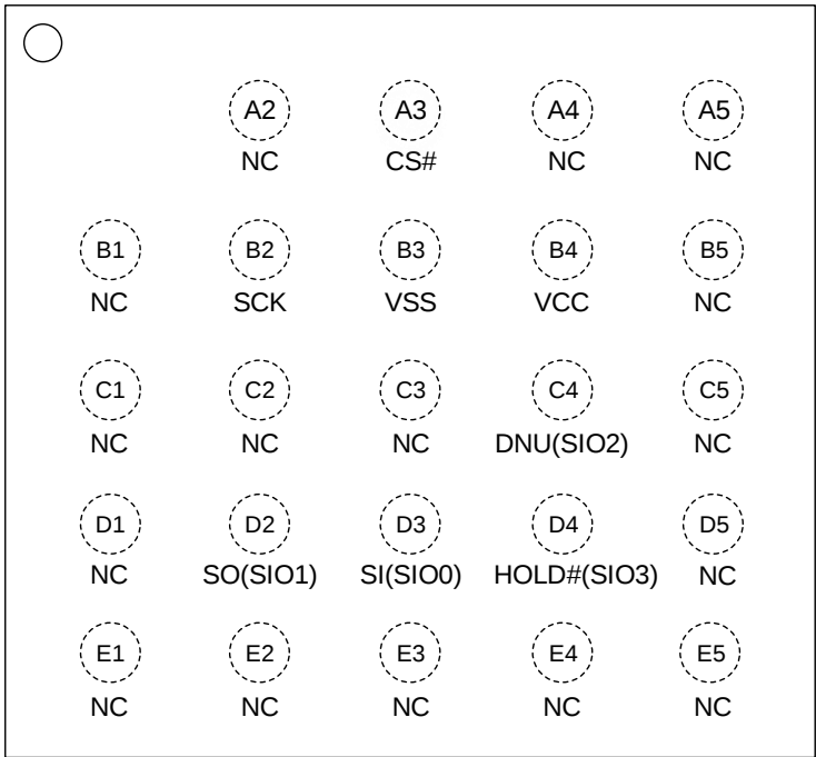
24-ball TFBGA
