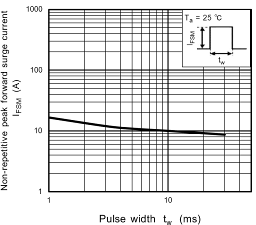
Fig. 8.5 I_{FSM} - t_w
