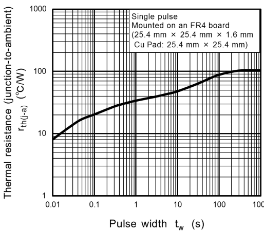
Fig. 8.4 r_{th} - t_w
