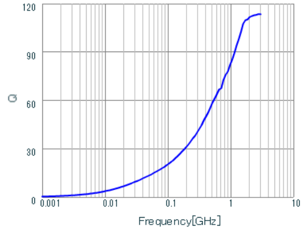
LQW15AN3N0B80 Q.
