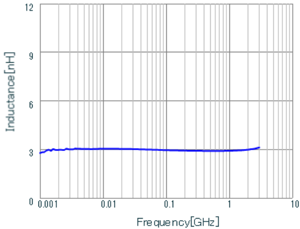
LQW15AN3N0B80 L.
