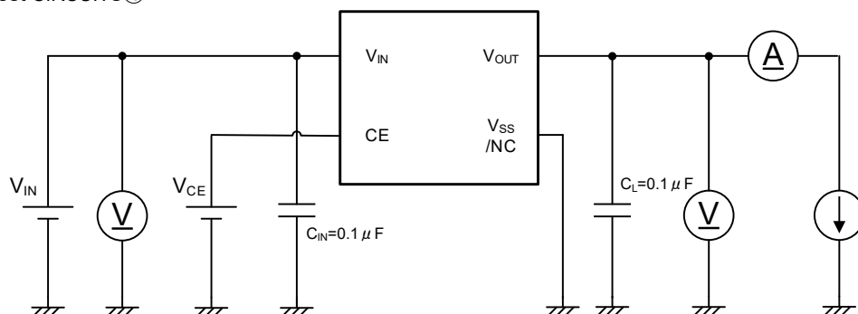
Test CIRCUITS④
