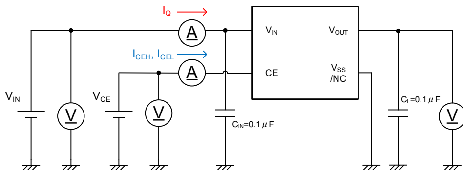
Test CIRCUITS①
