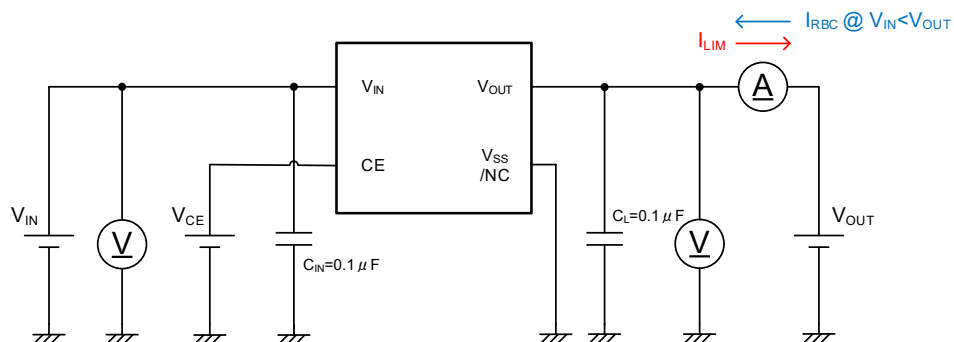
Test CIRCUITS③
