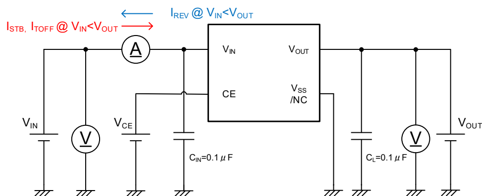
Test CIRCUITS②
