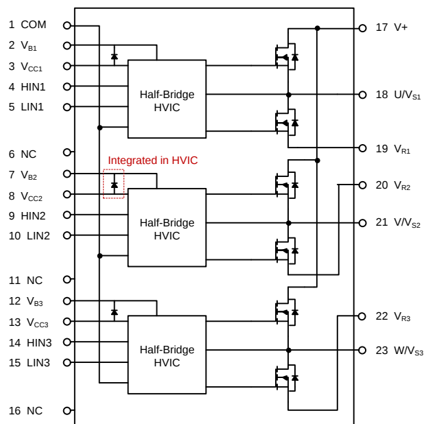
IRSM515-065
