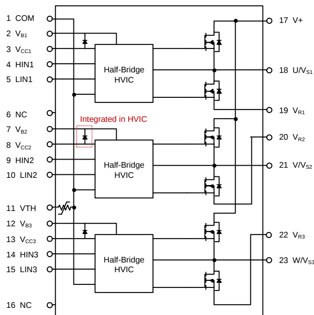
IRSM505-065
