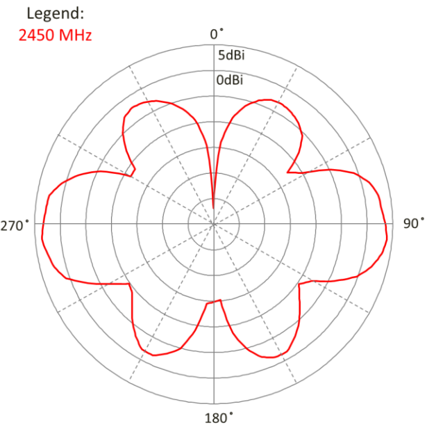
Elevation 2
