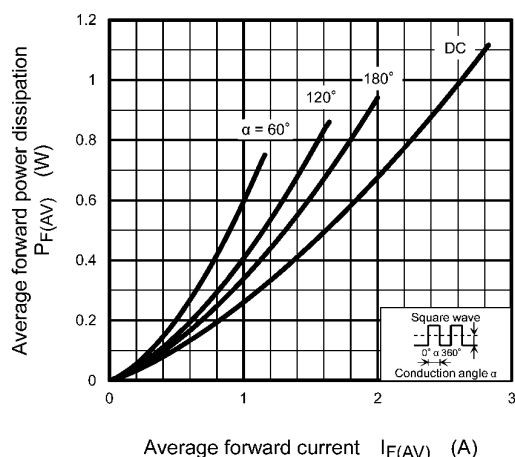
Fig. 10.2 P_{F(AV)} - I_{F(AV)}
