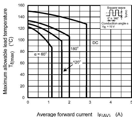
Fig. 10.4 T_{t(max)} - I_{F(AV)}
