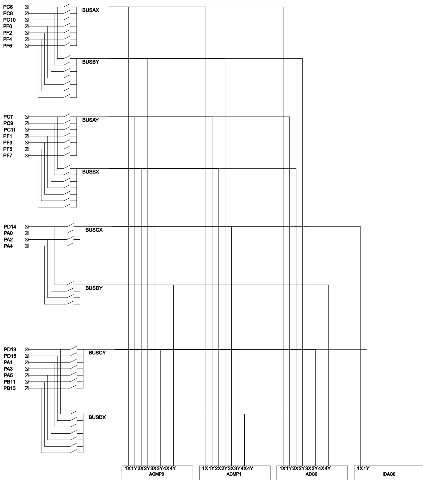
Figure 7.2. ARTIK 020 APORT
