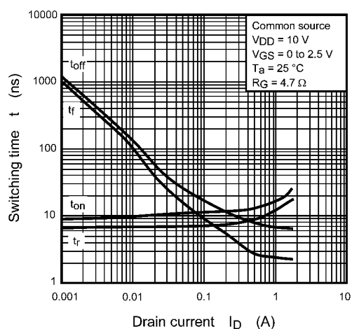
Fig. 7.11 t - I_D
