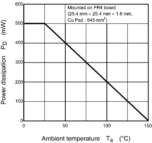
Fig. 7.14 P_D - T_a
