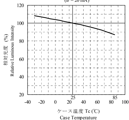
相対光度 — ケース温度特性 Relative Luminous Intensity vs. Case Temperature ( I_f = 20\text{ mA} )
