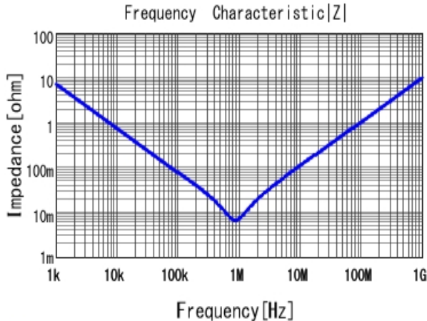
■ ECASD41E226M040KA0 |Z| DCOV, 25degC
