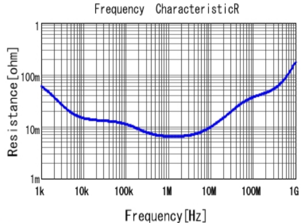
■ ECASD41E226M040KA0 R DCOV, 25degC
