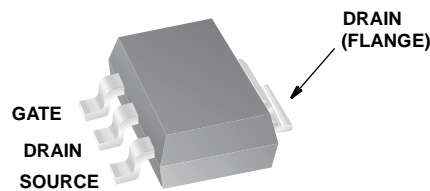
SOT-223
