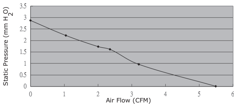
CFM-4010B-065-251
