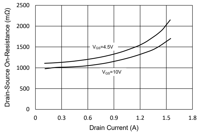
Fig.4 - R_{DS(ON)} - I_D
