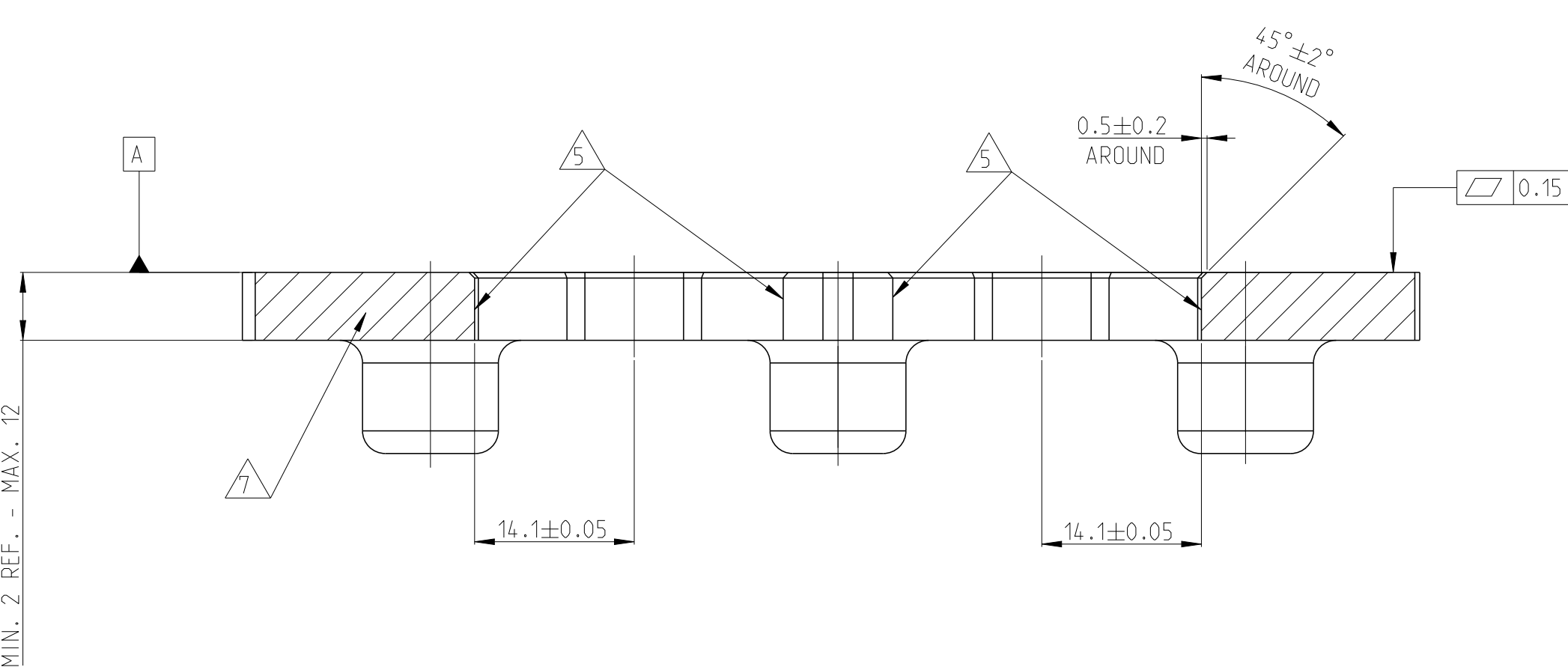
SECTION A-A
