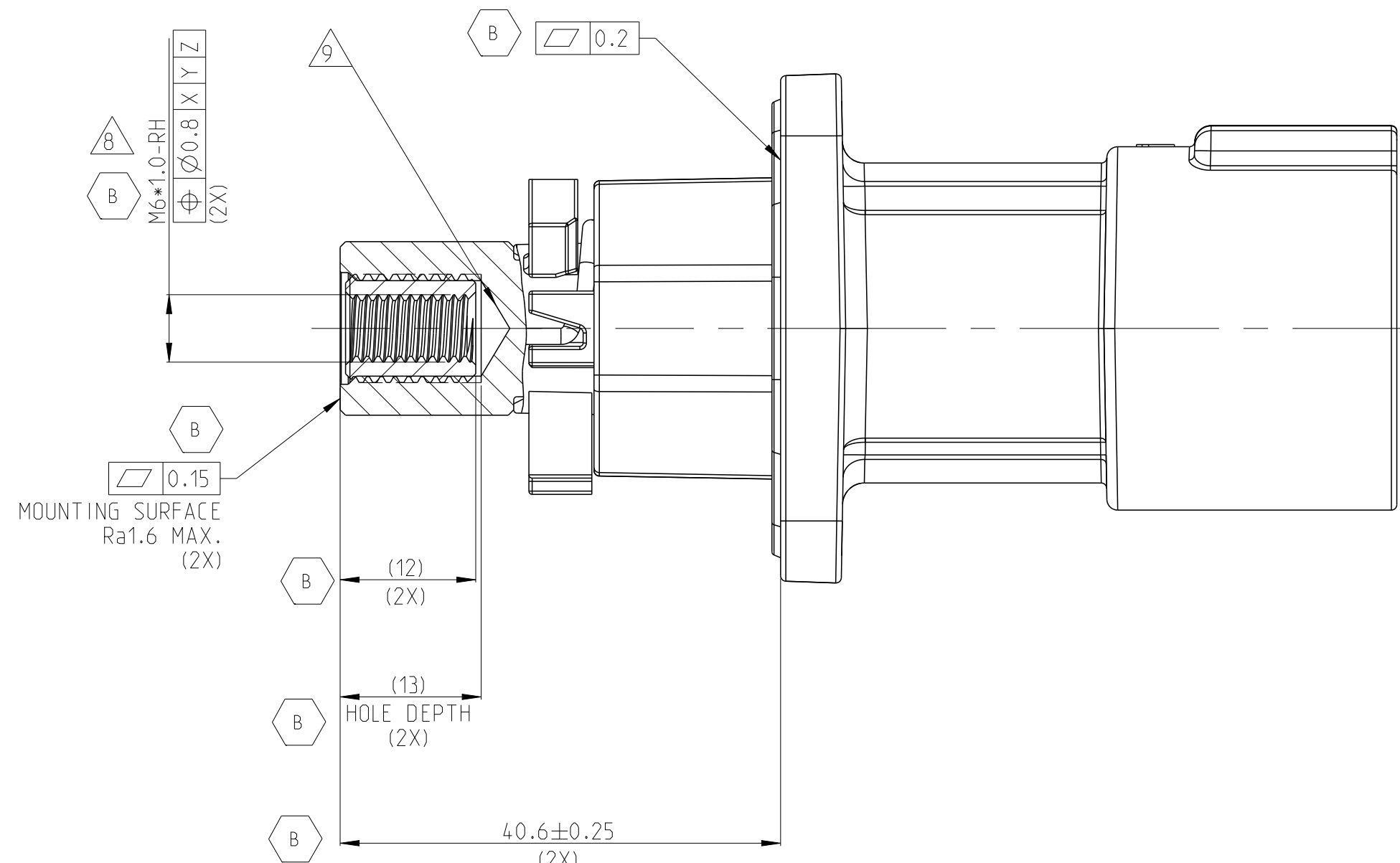
SECTION A-A
