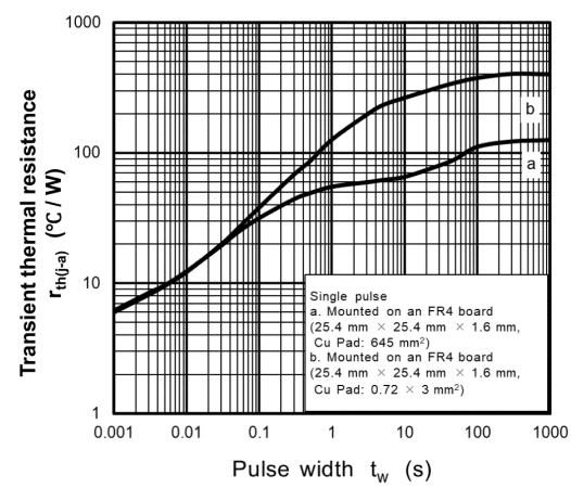
Fig. 8.11 r_{th(j-a)} - t_w
