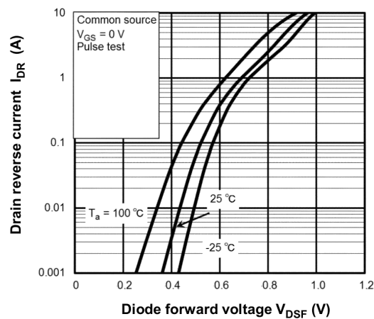
Fig. 8.7 I_{DR} - V_{DSF}
