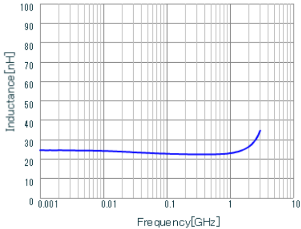
LQW15AN23NG80 L.
