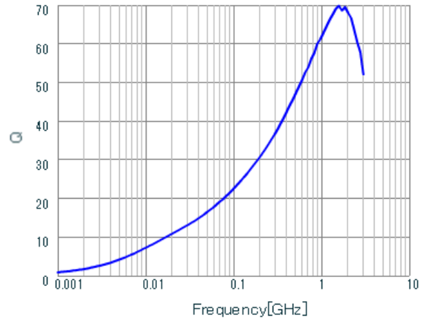
LQW15AN23NG80 Q.
