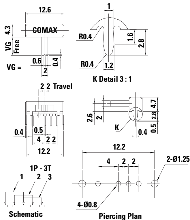
SK-13D16-VG 5 PA 1P3T 5mm Knob
