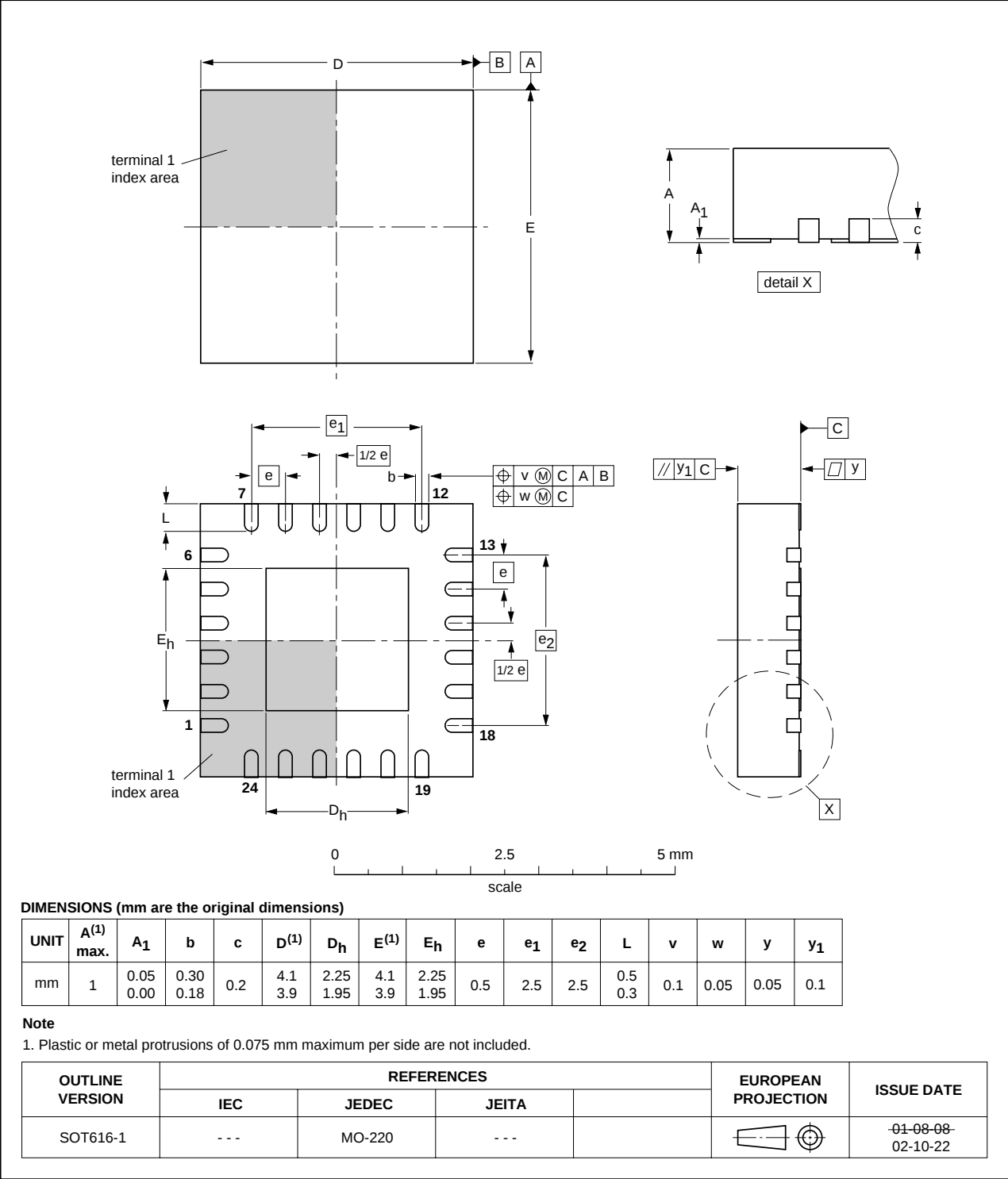
Fig 29. Package outline SOT616-1
