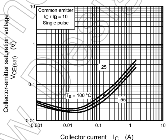
Fig. 7.4 V_{CE(sat)} - I_C
