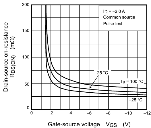
Fig. 8.2.3 R_{DS(ON)} - V_{GS}
