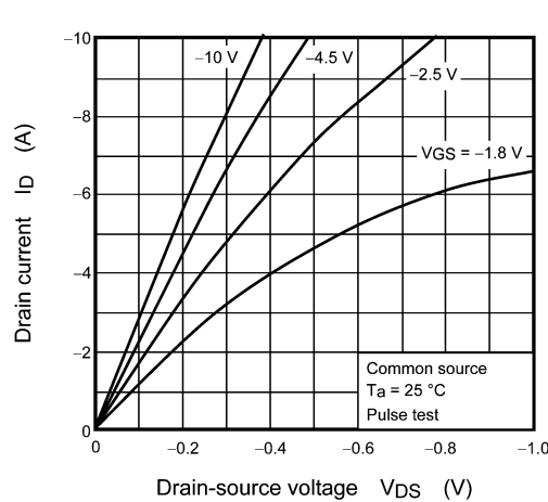
Fig. 8.2.1 I_D - V_{DS}
