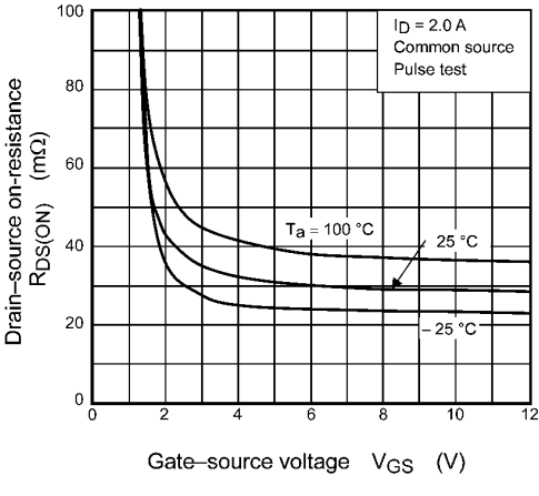
Fig. 8.1.4 R_{DS(ON)} - V_{GS}
