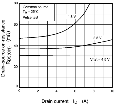
Fig. 8.1.5 R_{DS(ON)} - I_D
