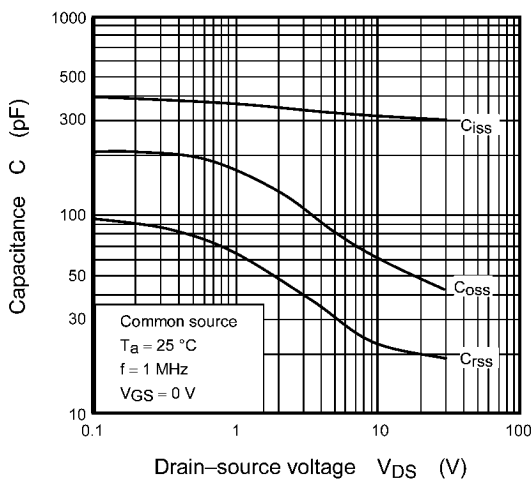
Fig. 8.1.9 C - V_{DS}
