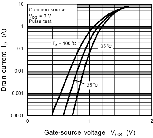
Fig. 8.1.2 I_D - V_{GS}
