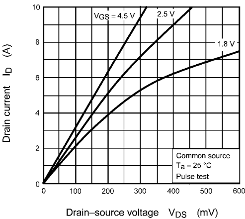
Fig. 8.1.1 I_D - V_{DS}
