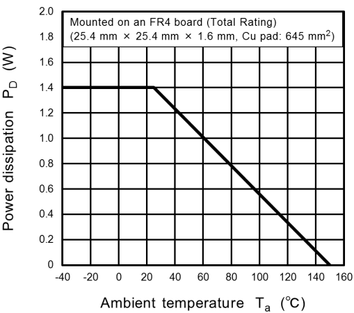
Fig. 8.3.2 P_D - T_a
