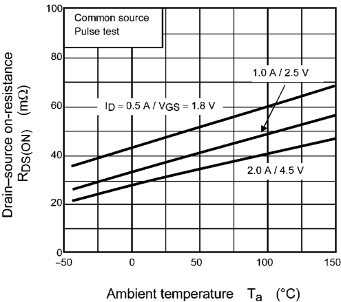
Fig. 8.1.6 R_{DS(ON)} - T_a
