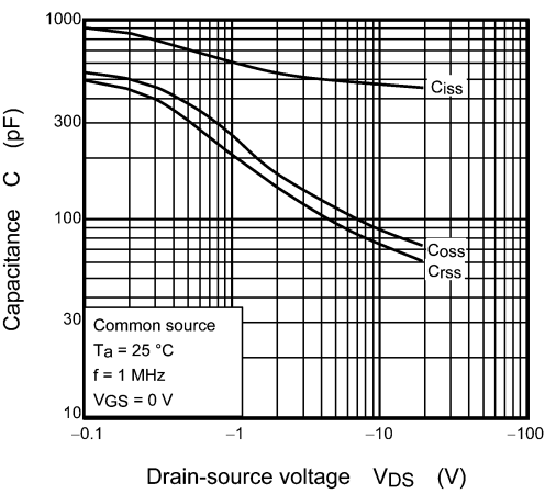
Fig. 8.2.8 C - V_{DS}
