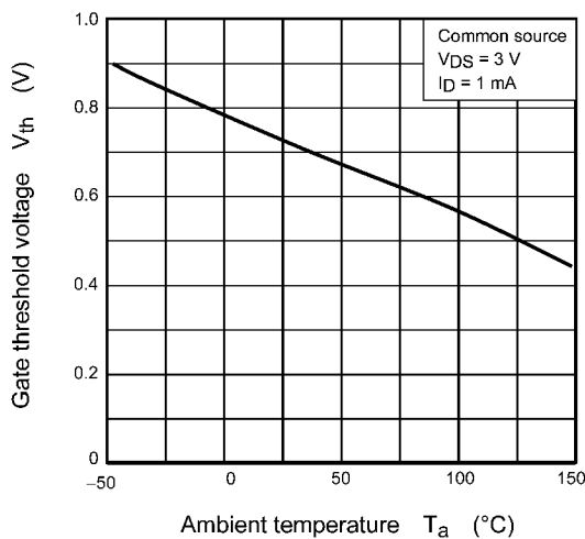
Fig. 8.1.7 V_{th} - T_a
