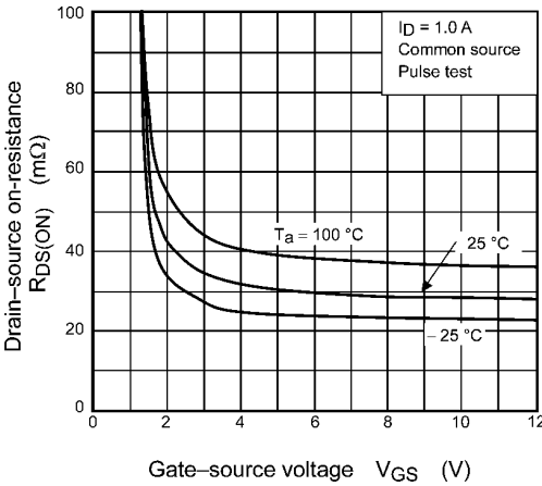
Fig. 8.1.3 R_{DS(ON)} - V_{GS}
