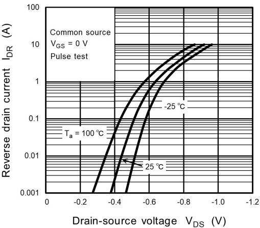
Fig. 8.1.8 I_{DR} - V_{DS}
