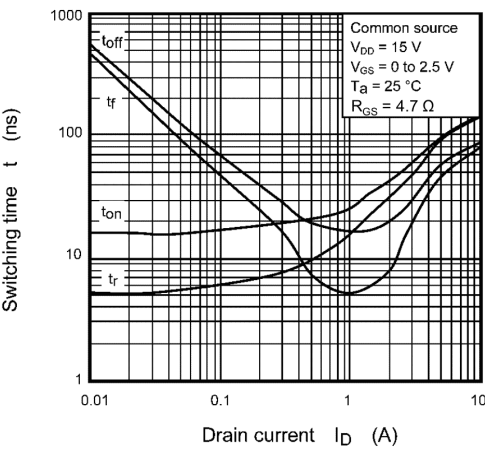
Fig. 8.1.10 t - I_D
