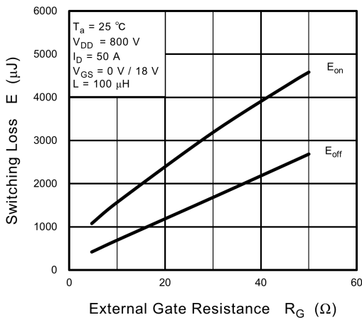
Fig. 8.16 E - R_G
