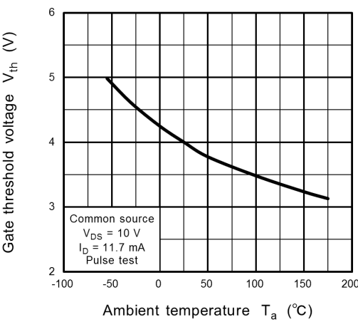
Fig. 8.4 V_{th} - T_a
