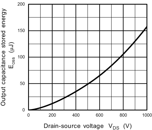
Fig. 8.14 E_{oss} - V_{DS}
