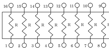
独立回路 / Isolated Circuit TSN3A
