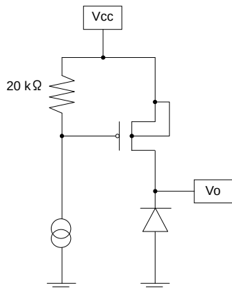
Vo Pin
