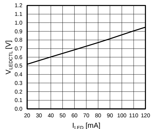
Figure 17. V_{\text{LEDCTL}} vs I_{\text{LED}}
