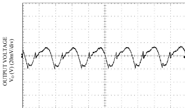
Vo=1.8V, Io = Io,max, Vin=12V
