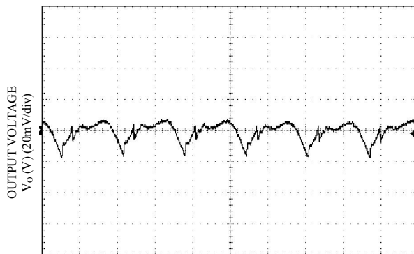
Vo=1.8V, Io = Io,max, Vin=12V
