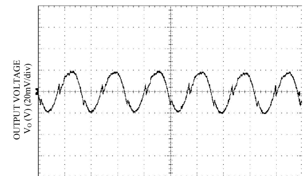
Vo=2.5V, Io = Io,max, Vin=12V
