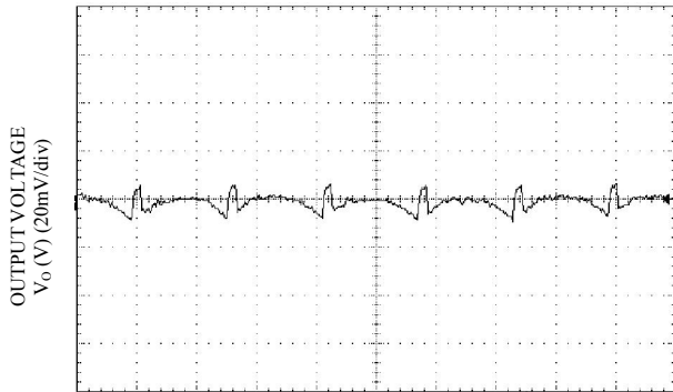
Vo=0.6V, Io = Io,max, Vin=8V
