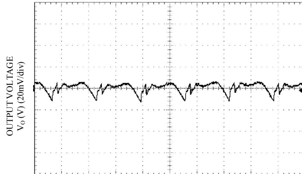
Vo=1.2V, Io = Io,max, Vin=12V
