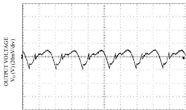
Vo=1.2V, Io = Io,max, Vin=12V
