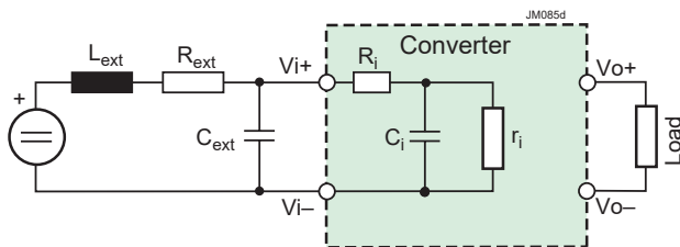
Fig. 2 Input configuration
