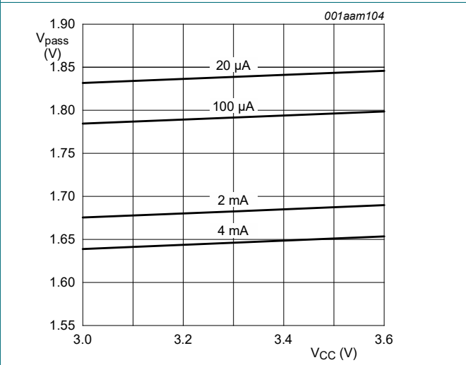
Fig. 9. Pass voltage versus supply voltage; T amb = 25 °C (typical)
