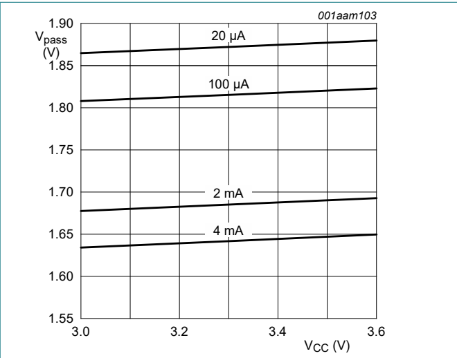
Fig. 8. Pass voltage versus supply voltage; T amb = 85 °C (typical)
