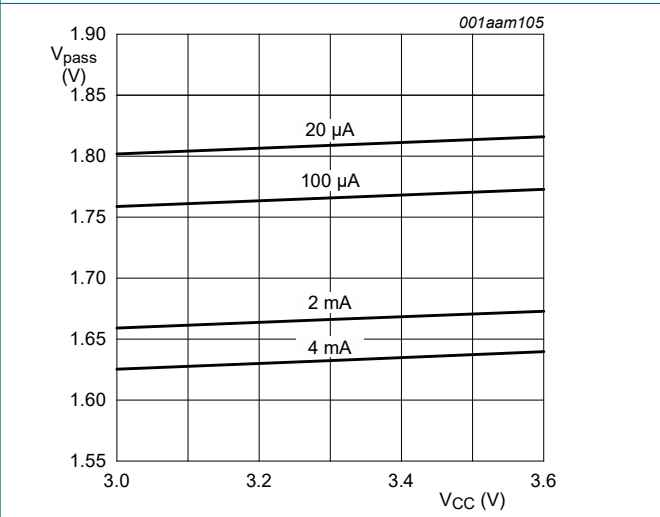
Fig. 10. Pass voltage versus supply voltage; T amb = 0 °C (typical)
