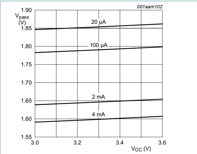
Fig. 7. Pass voltage versus supply voltage; T amb = 125 °C (typical)
