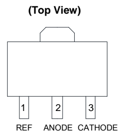
SOT89 (Option 1)
