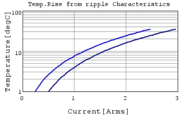
GRM155C80J105KE15 Temp.rise — 500kHz —
