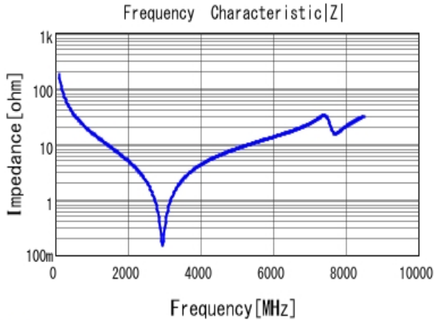
■ GCQ1555C1H8R9DB01 |Z| DC0V, 25degC
