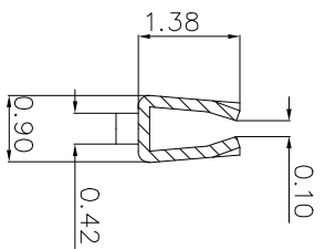
SECTION: C-C SCALE: 1:1
