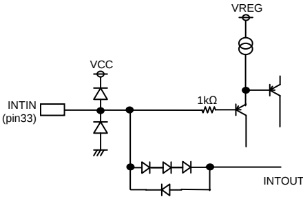
○ INTIN pin
