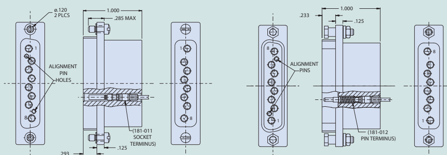
180-066 Plug
