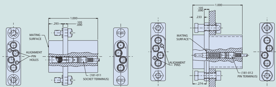
180-064 Plug
