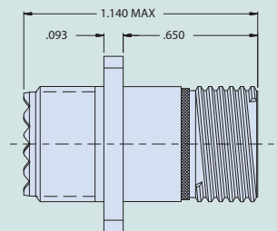
07- Wall Mount Receptacle
