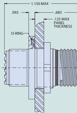
08- Jam Nut Receptacle
