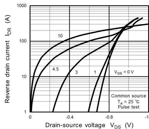
Fig. 8.6 I_{DR} - V_{DS}
