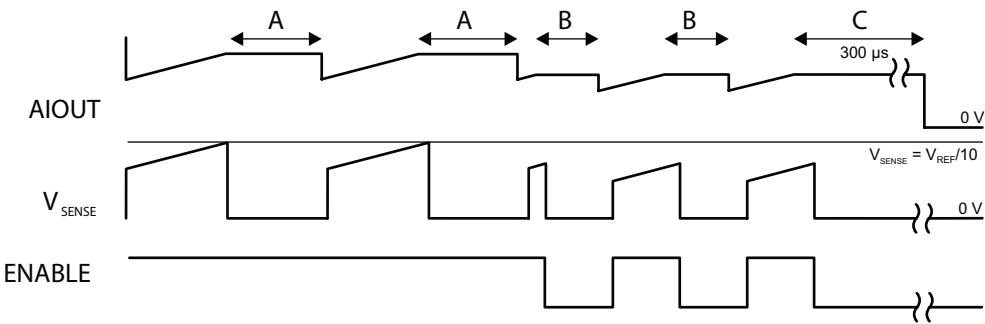
AIOUT Output
