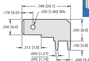
.250 (6.4) TAB
