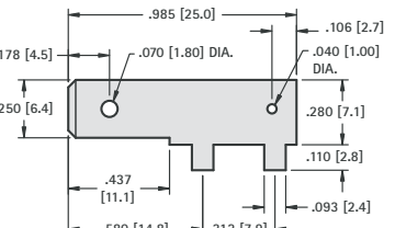
.250 (6.4) TAB
