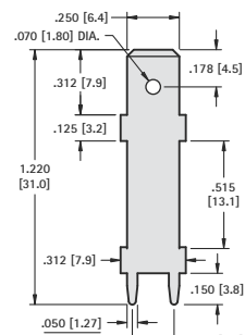
.250 (6.4) TAB
