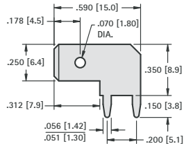
.250 (6.4) TAB
