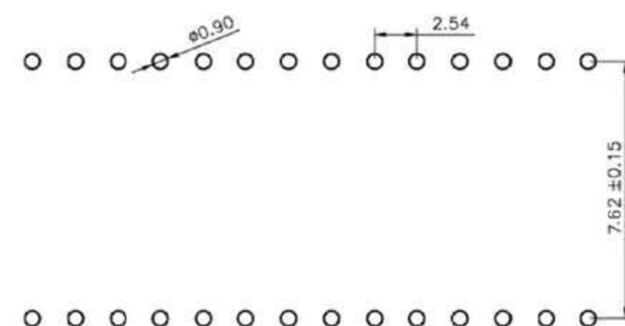
P.C.B LAYOUT
